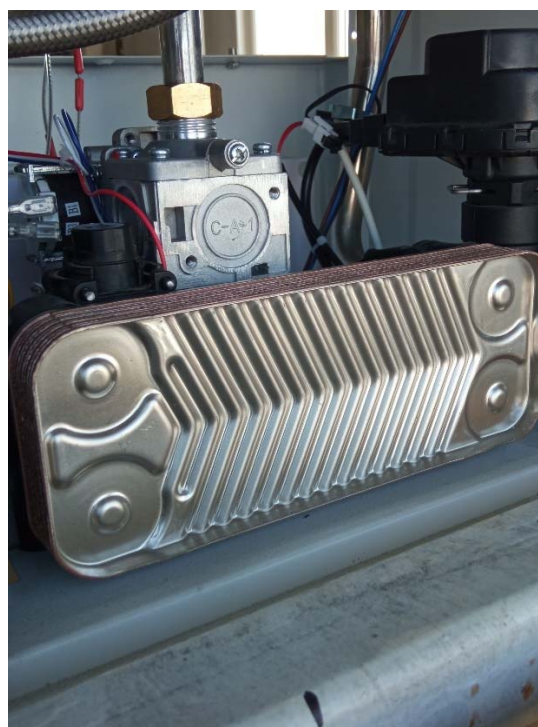
Рис.2 Вторичный пластинчатый теплообменник ГВС из нержавеющей стали
