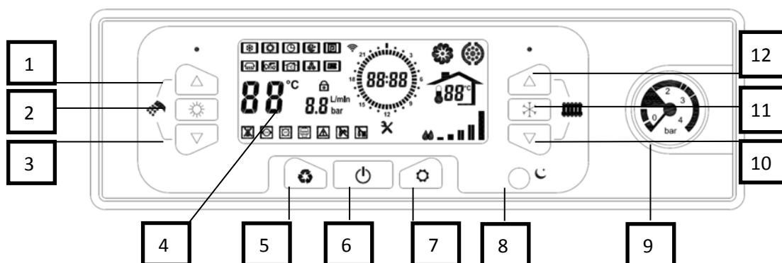
Рис.17 Панель управления
