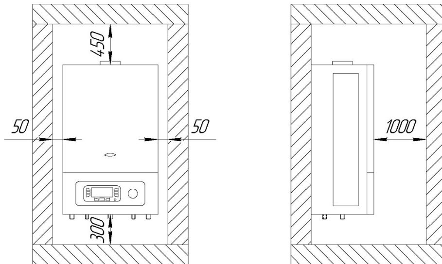
Рис.19 Минимально допустимые расстояния от котла при монтаже
