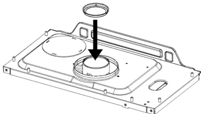
Рис. 18 Схема установки диафрагмы на котел
