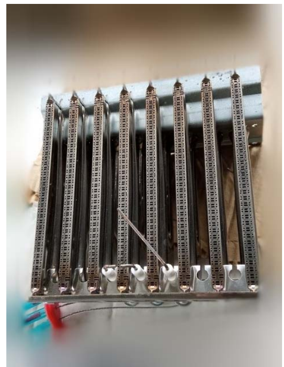
Рис.10 Газовая горелка с насадками (ламелями), двумя электродами розжига и электродом контроля пламени
