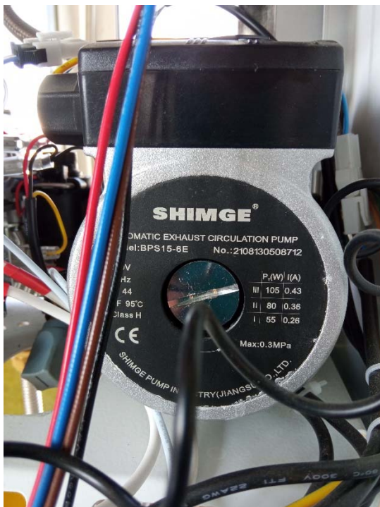
Рис. 5 Циркуляционный насос
